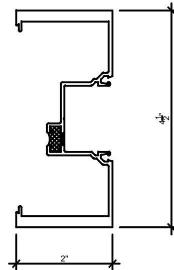
8 HEAVY VERTICAL SCALE: 6" = 1'-0"
