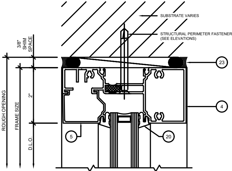
1 SF300T OPTIONAL HEAD 5 SCALE: 6" = 1'-0"
