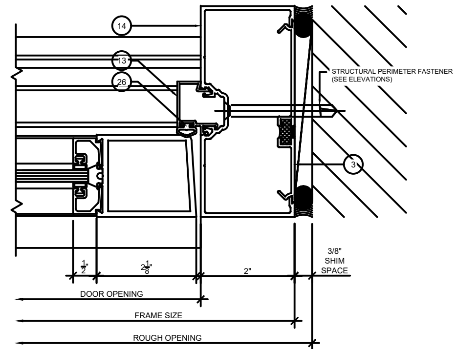
3 SF300T DOOR JAMB 6 SCALE: 6" = 1'-0"
