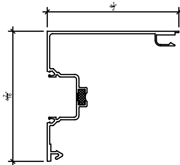
11 CORNER POST SCALE: 6" = 1'-0"
