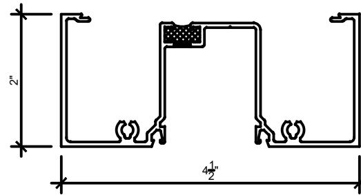
2 DEEP POCKET MULLION SCALE: 6" = 1'-0"
