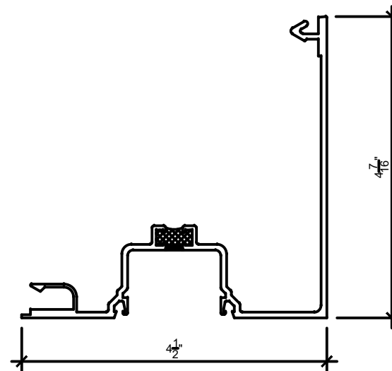
12 CORNER POST SCALE: 6" = 1'-0"
