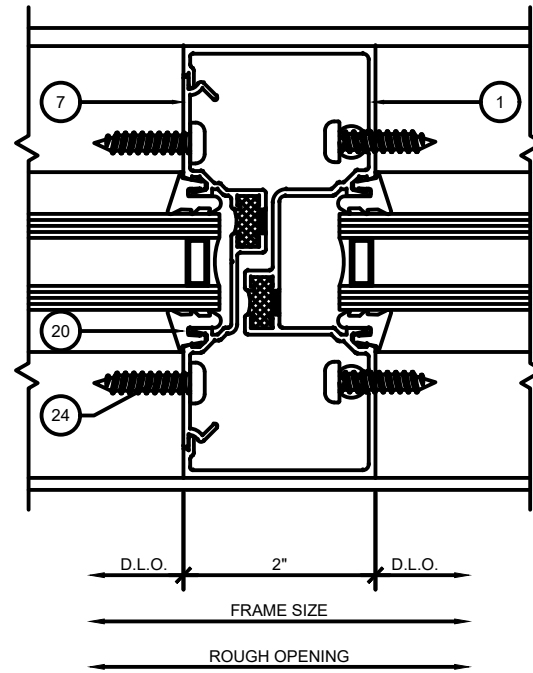
4 SF300T VERTICAL 3 SCALE: 6" = 1'-0"
