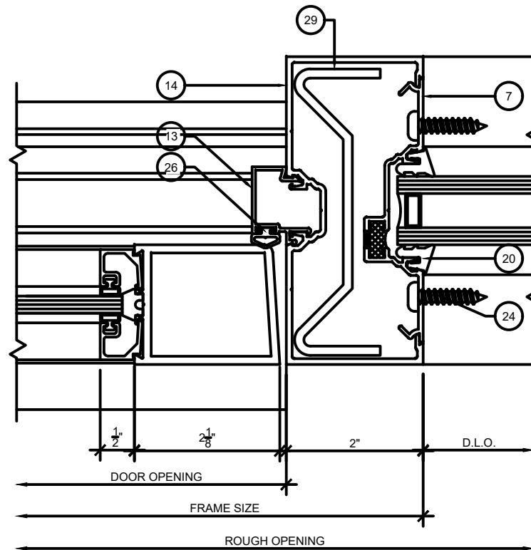
2 SF300T DOOR SIDELITE 6 SCALE: 6" = 1'-0"
