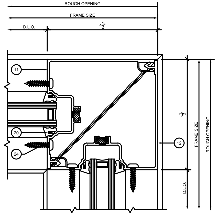
3 7 SF300T 90° CORNER POST SCALE: 6" = 1'-0"
