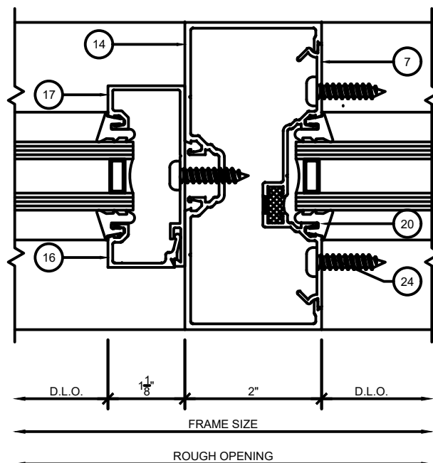
4 SF300T TRANSOM SIDELITE 6 SCALE: 6" = 1'-0"
