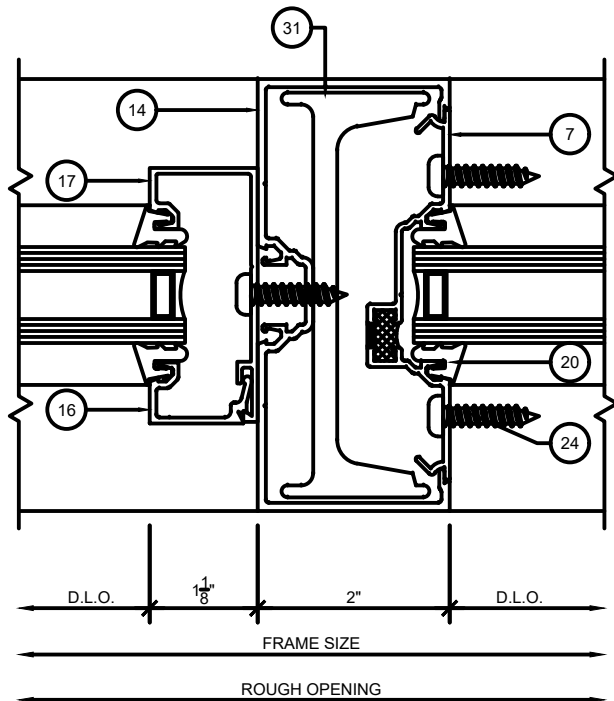
1 7 SF300T DOOR SIDELITE SCALE: 6" = 1'-0"
