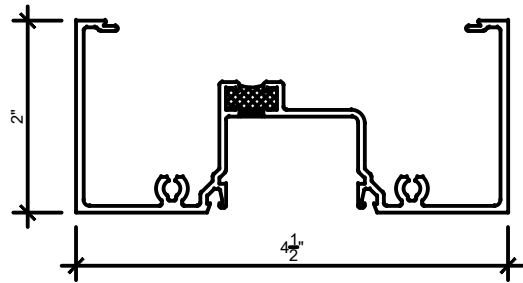
1 HEAD/VERTICAL SCALE: 6" = 1'-0"
