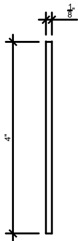
26 GASKET SCALE: 1'-0" = 1'-0"
