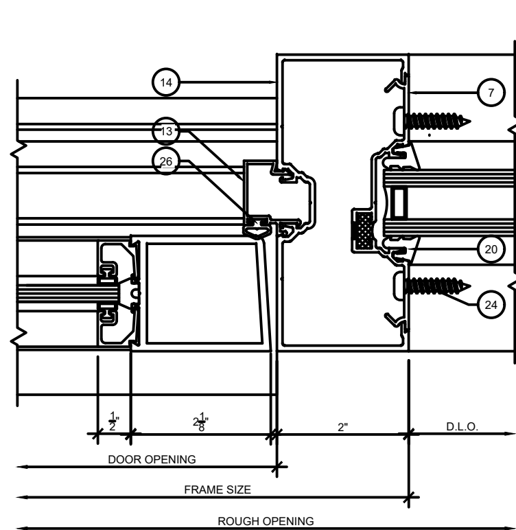
1 SF300T DOOR SIDELITE 6 SCALE: 6" = 1'-0"
