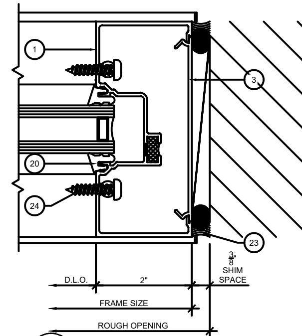
6 SF300T JAMB 3 SCALE: 6" = 1'-0"
