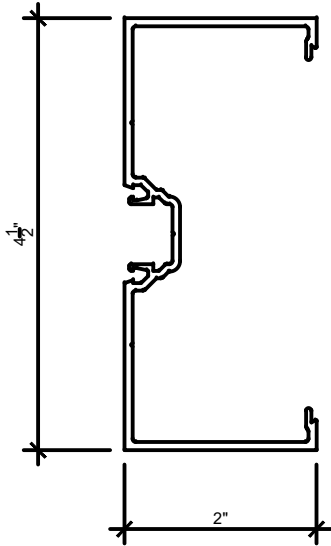
14 DOOR JAMB SCALE: 6" = 1'-0"
