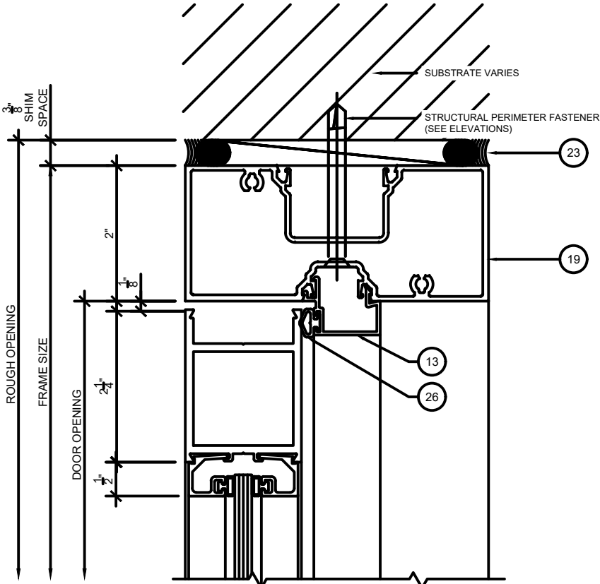
3 SF300T DOOR HEAD 5 SCALE: 6" = 1'-0"
