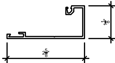
17 SASH SCALE: 6" = 1'-0"
