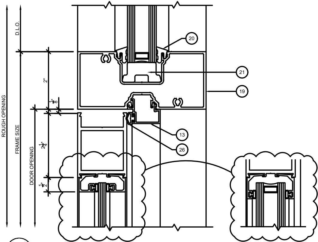
2 SF300T DOOR TRANSOM 5 SCALE: 6" = 1'-0"
