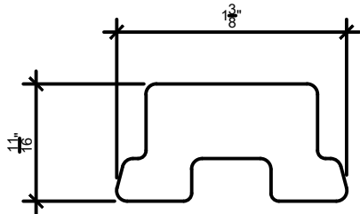
21 SETTING BLOCK SCALE: 1'-0" = 1'-0"
