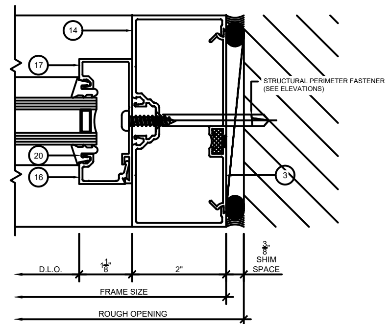
6 SF300T TRANSOM JAMB 6 SCALE: 6" = 1'-0"
