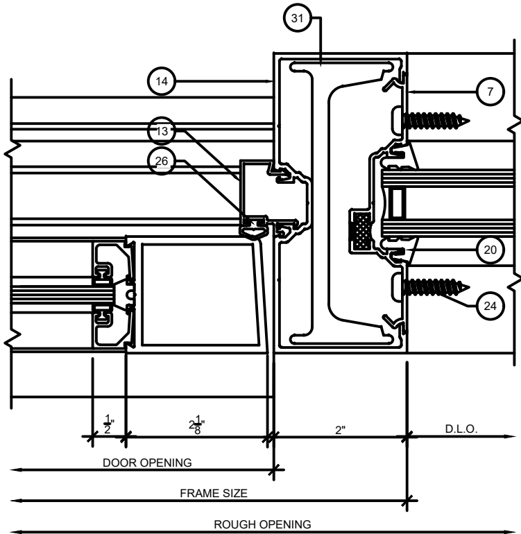
1 7 SF300T DOOR SIDELITE SCALE: 6" = 1'-0"
