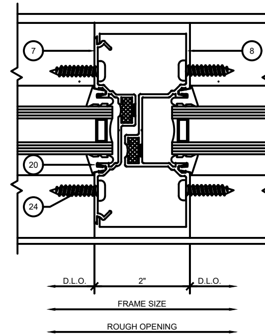
5 SF300T HEAVY VERTICAL 3 SCALE: 6" = 1'-0"
